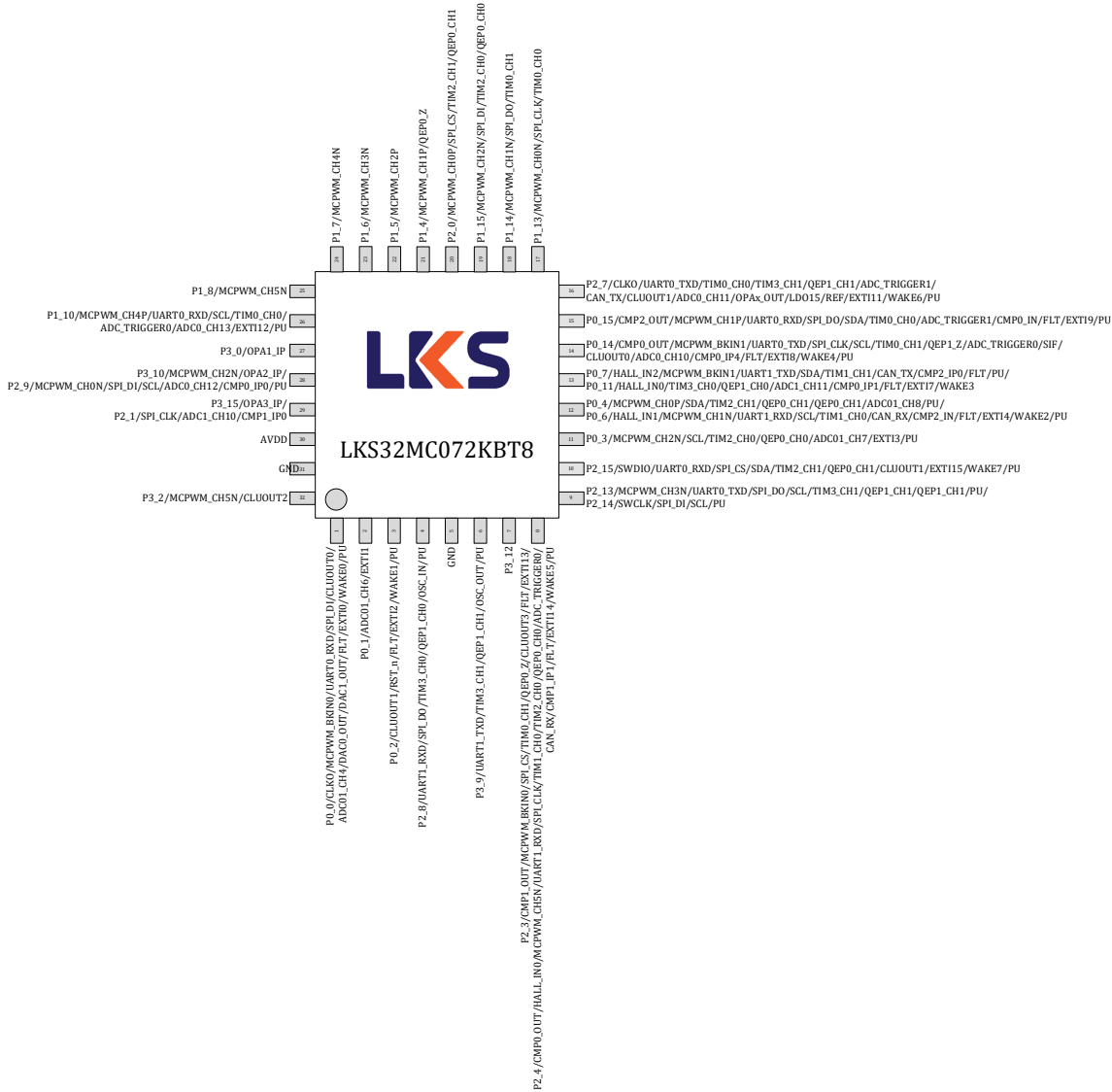
图 3-5 LKS32MC072KBT8 管脚分布图
