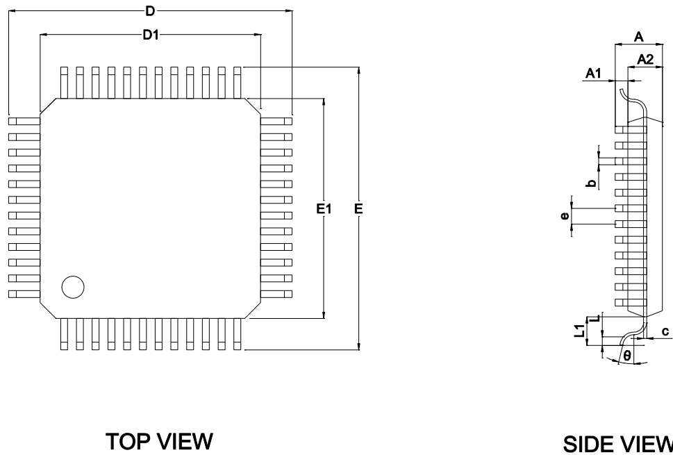
图 4-2 LKS32MC071CBT8/LKS32MC071C8T8 封装图示
