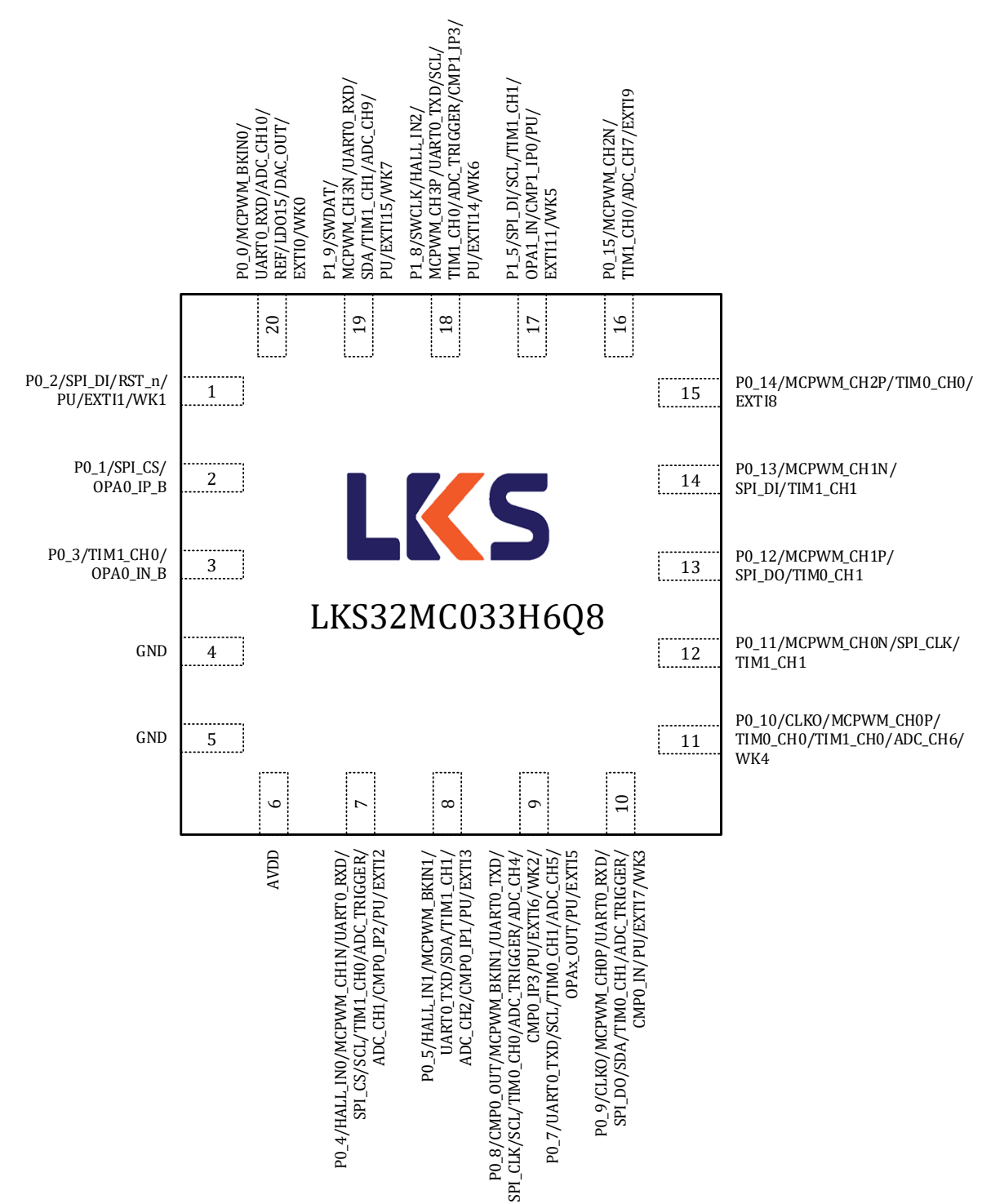
图 3-3 LKS32MC033H6Q8 管脚分布图
