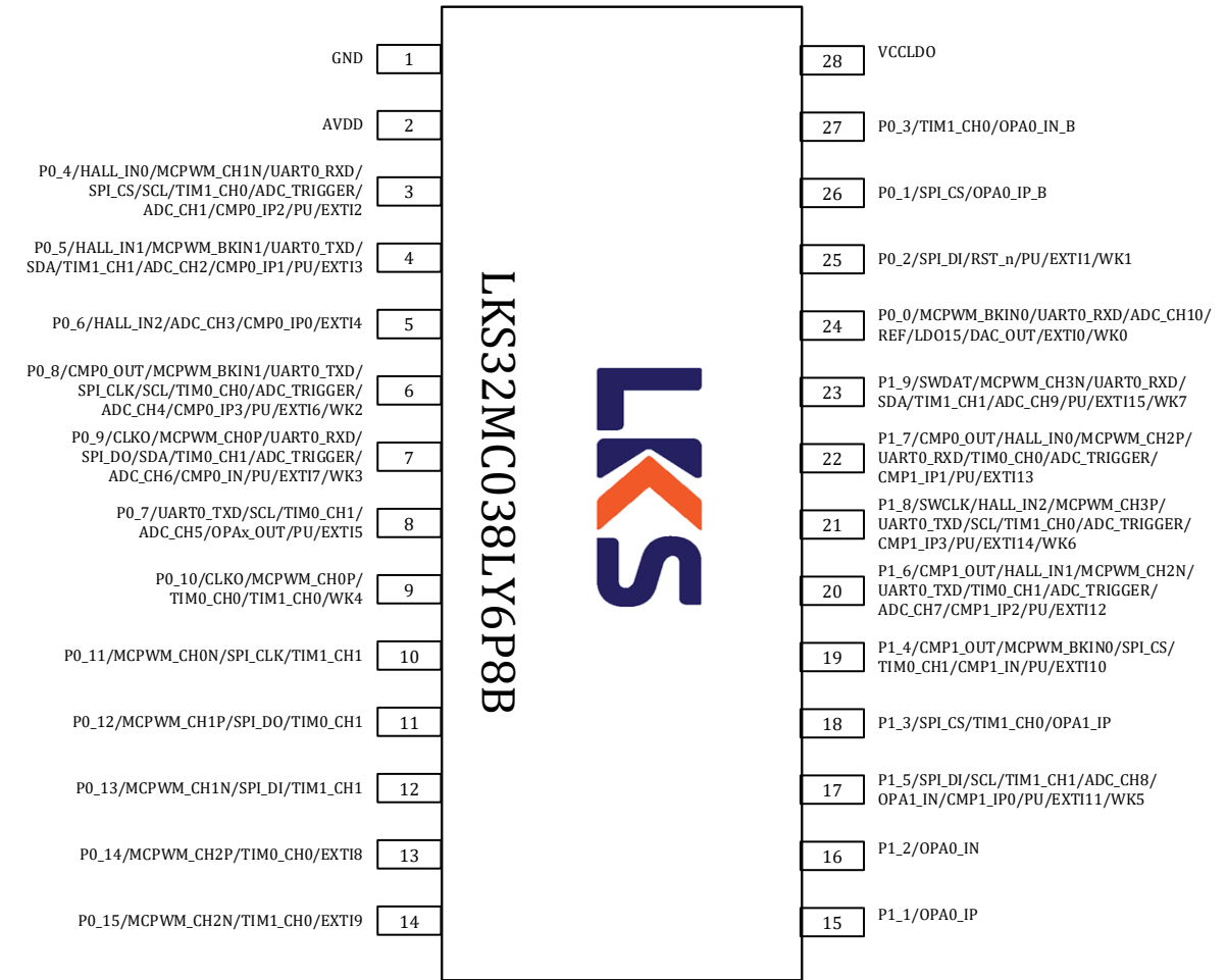
图 3-10 LKS32MC038LY6P8B/LKS32MC038LY6P8C 管脚分布图
