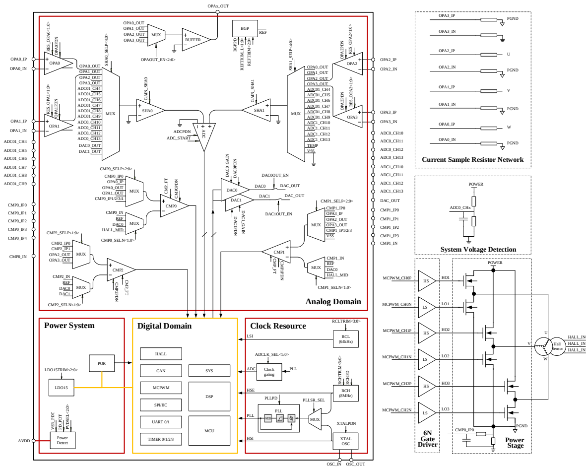
图 1-3 LKS32AT075 矢量正弦控制系统简化原理图
